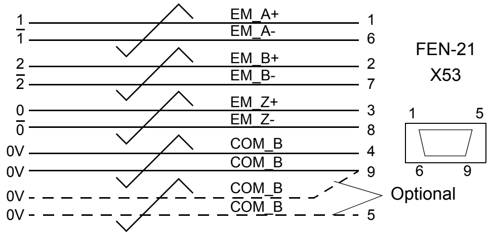
TTL encoder emulation output (X53)
