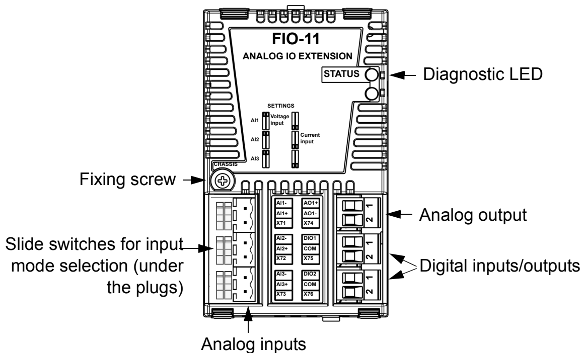
FIO-11 layout
